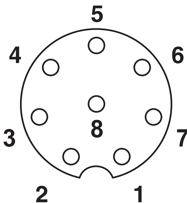
Schematisk ritning
