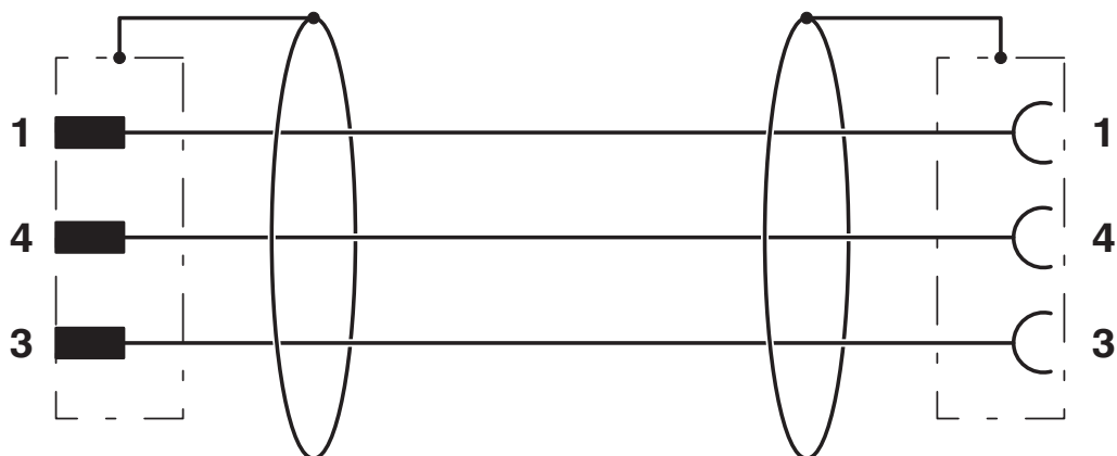
Anslutna M8-han-/honkontakter
