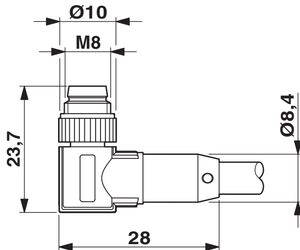
Måttskiss
