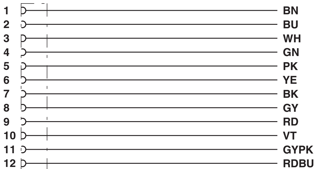
Anslutna M12-honkontakter
