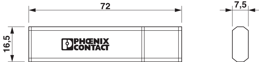
Måttskiss
