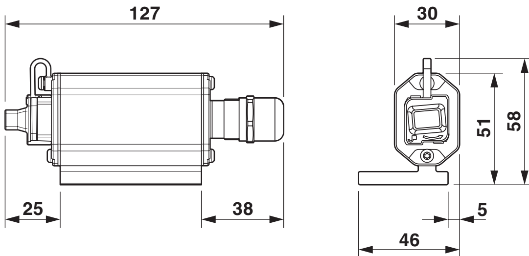
Måttskiss
