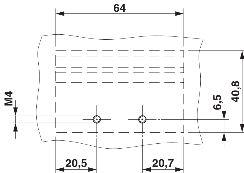
Borrplan/lödöns geometri
