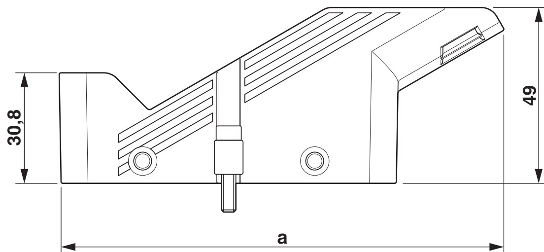
Måttskiss
