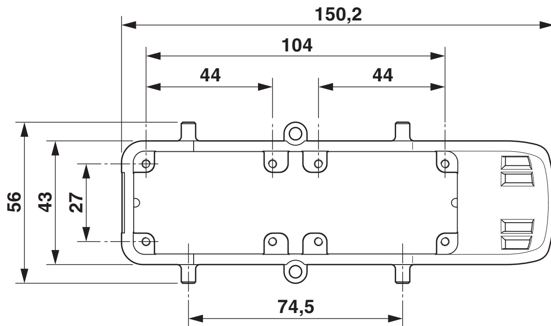
Måttskiss, vy uppifrån
