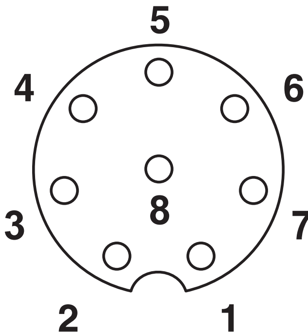
Schematisk ritning
