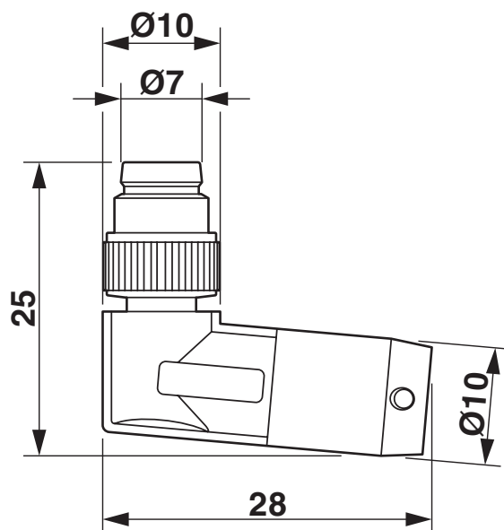
Måttskiss
