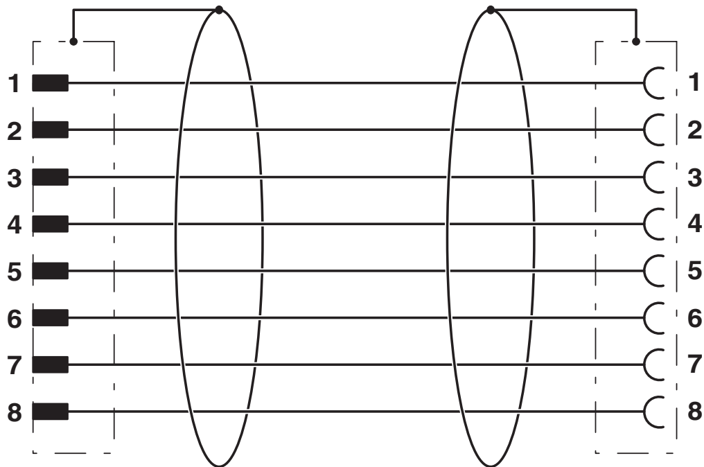
Kopplingsschema
