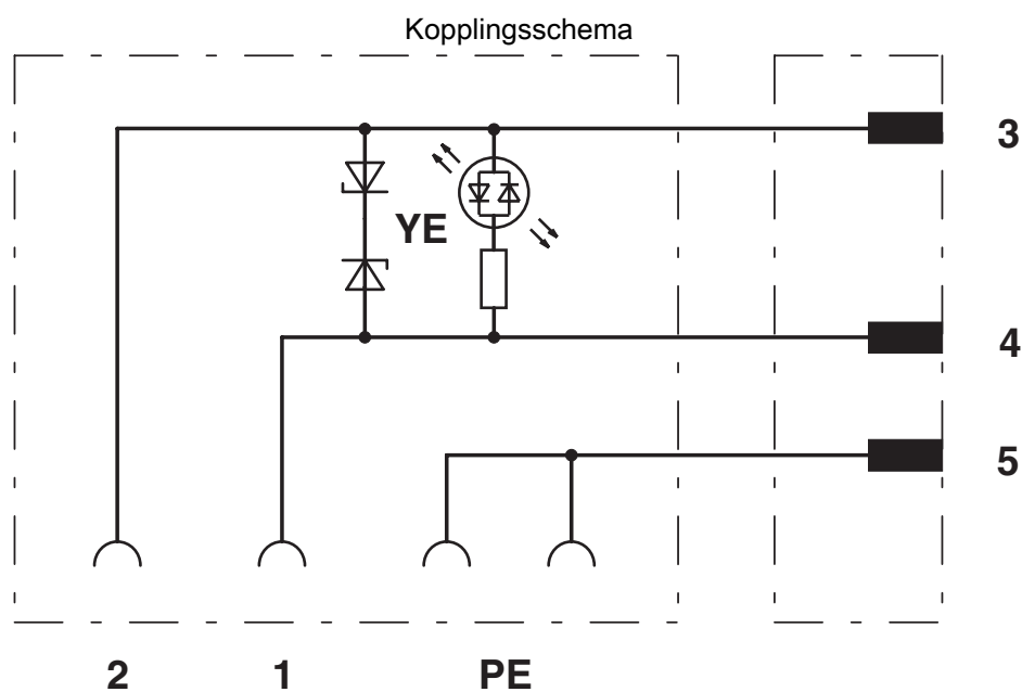
Anslutning av M12-hankontakten och ventilkontakten
