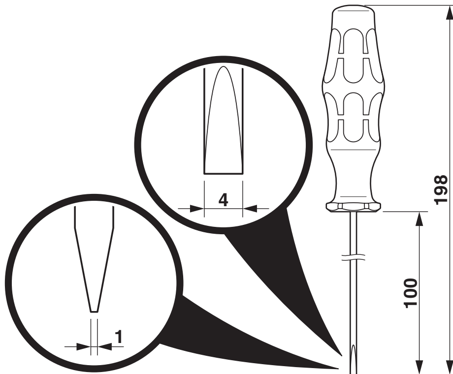
Måttskiss
