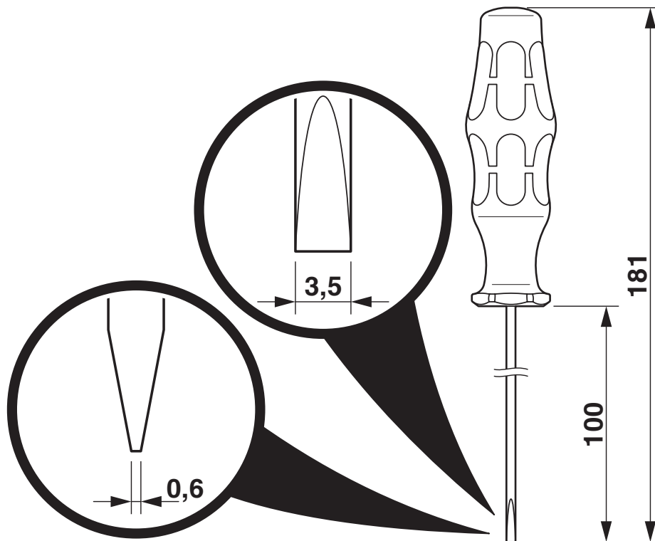
Måtskiss
