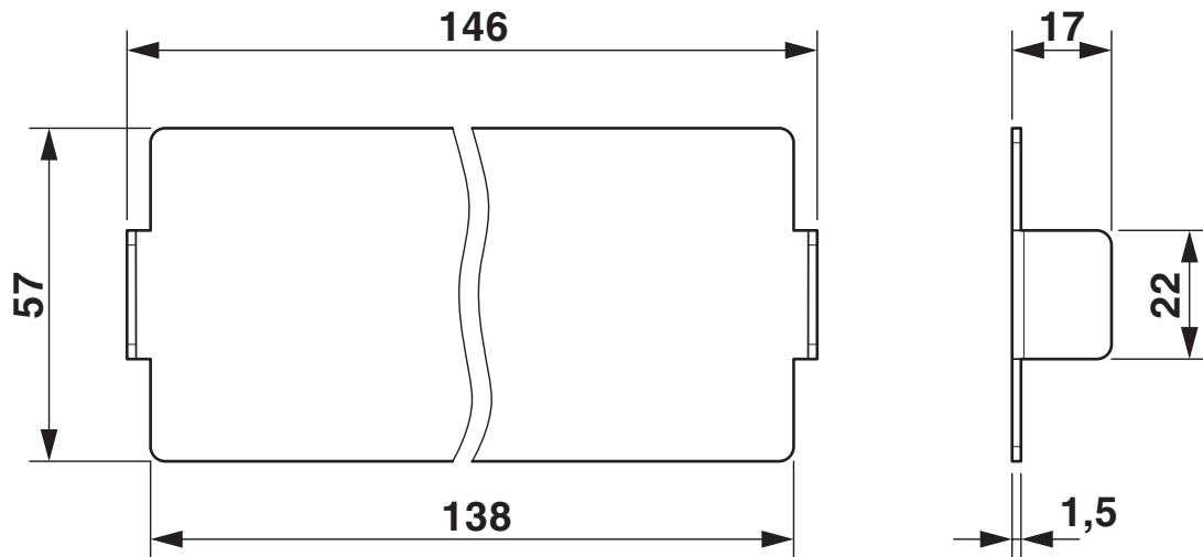
Måttskiss
