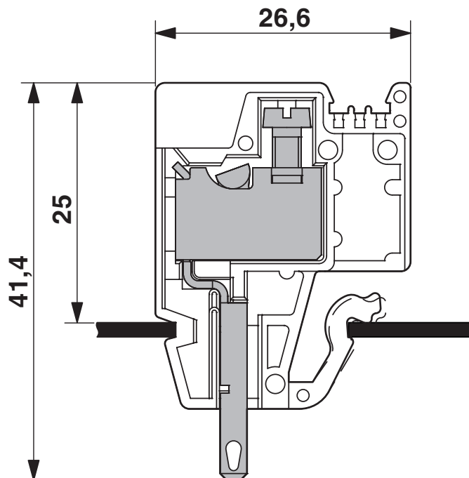
Måttskiss
