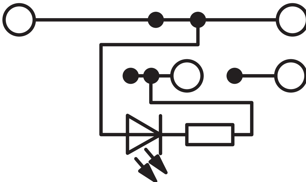
schakelschema
