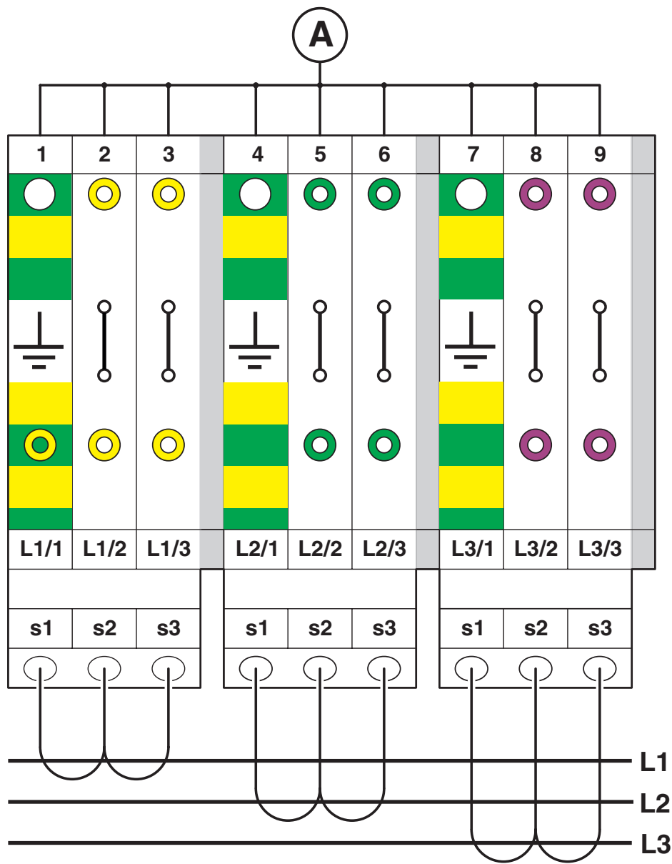
aansluitschema
