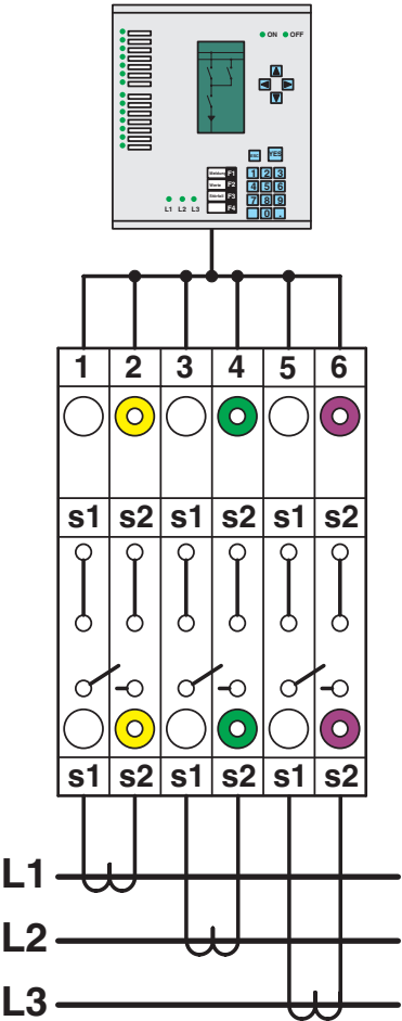
schematekening
