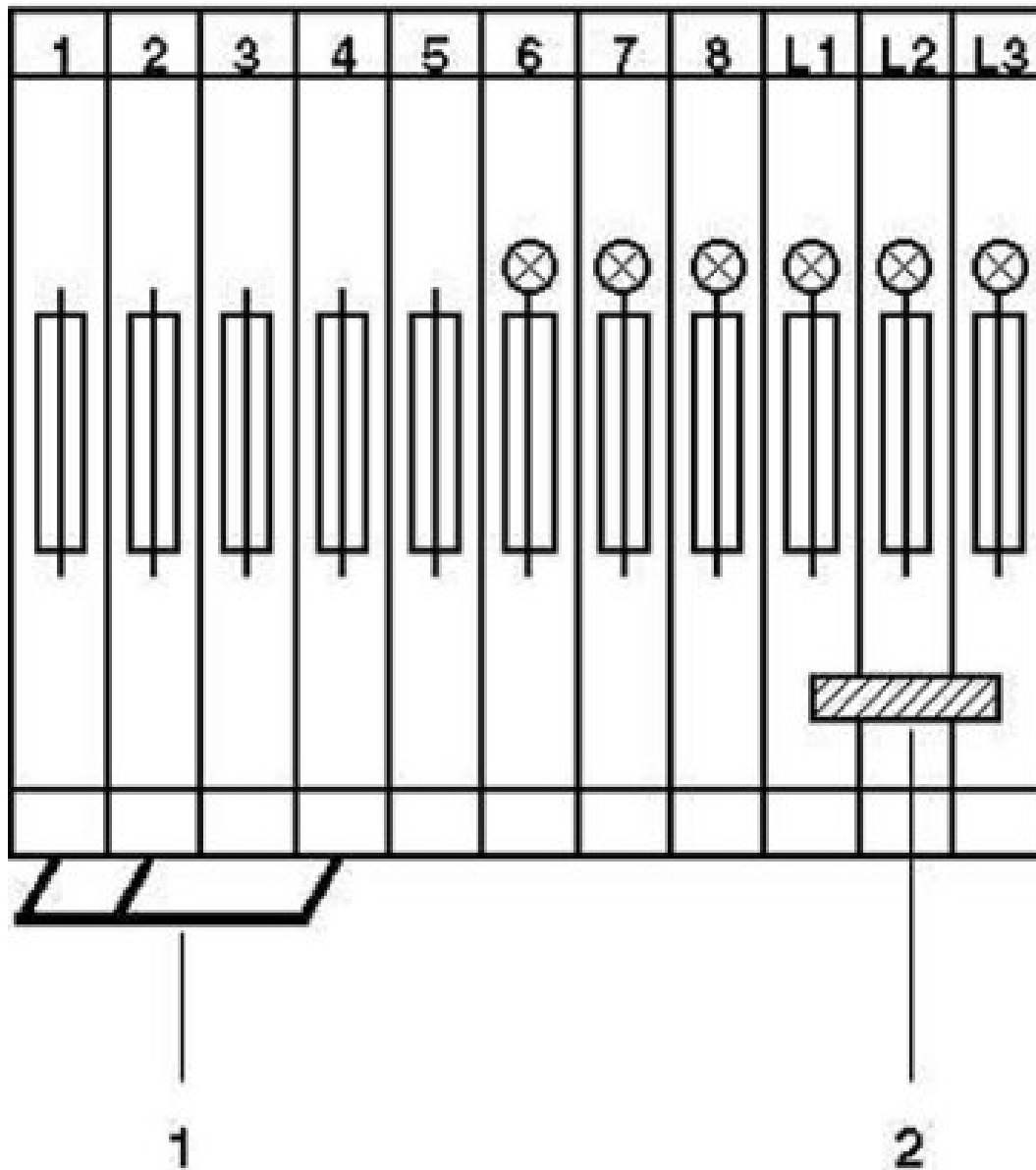
schakelschema
