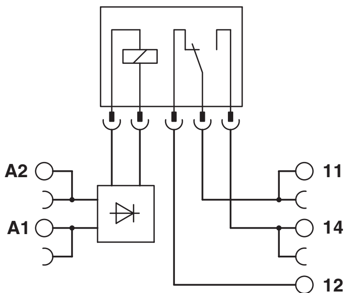
schakelschema
