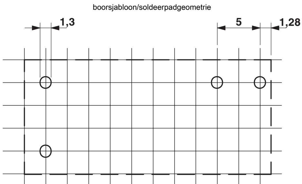
Aansluitschema: onderaanzicht
