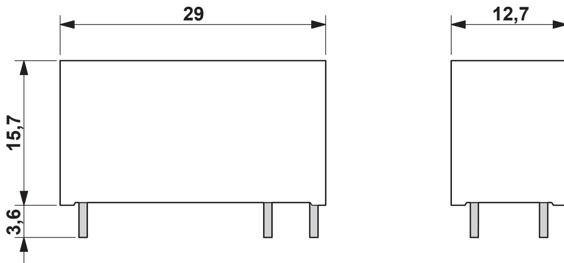
Maatschets
