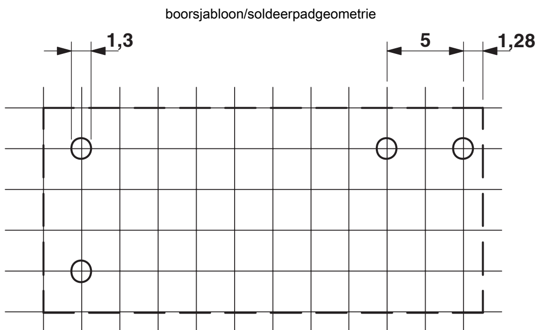
Aansluitschema: onderaanzicht
