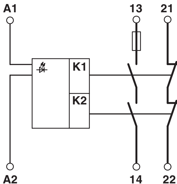
schakelschema
