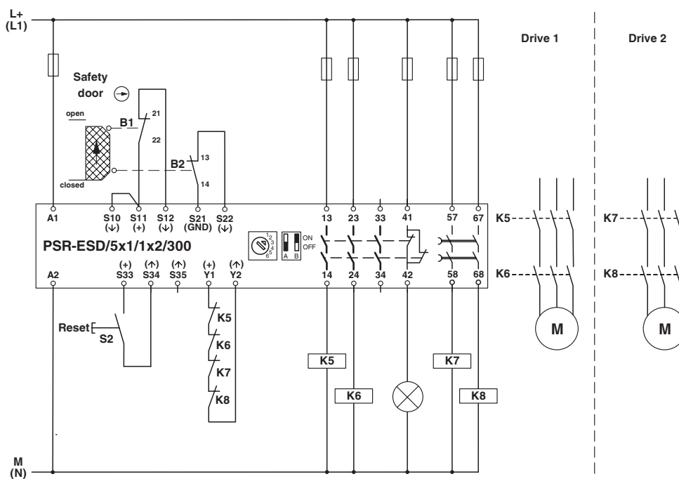
2-kanaals beveiligingsdeurbewaking
