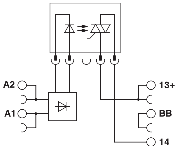
schakelschema
