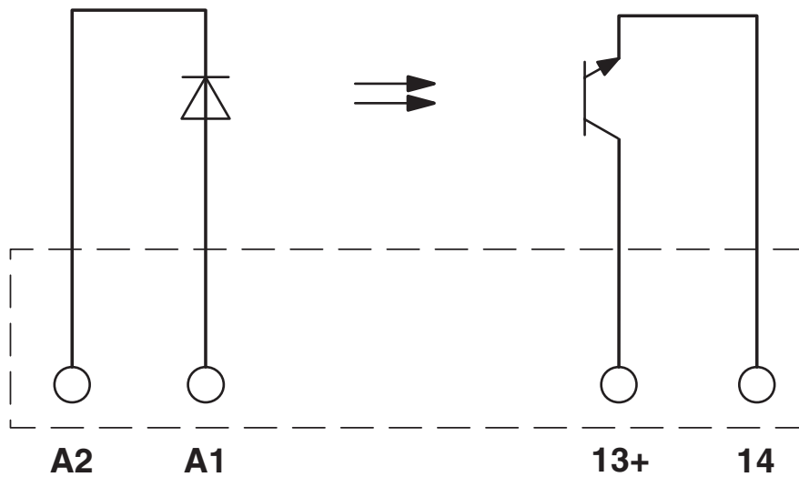
schakelschema
