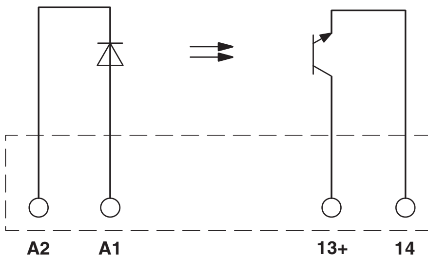
schakelschema
