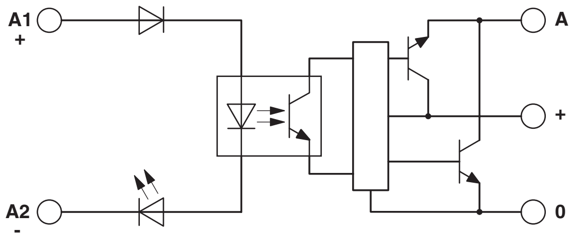
schakelschema
