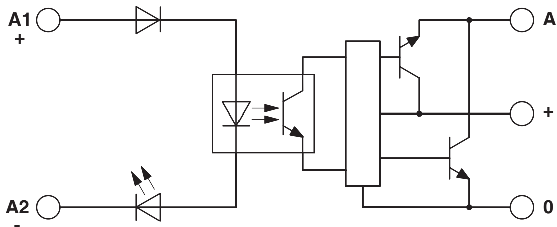
schakelschema
