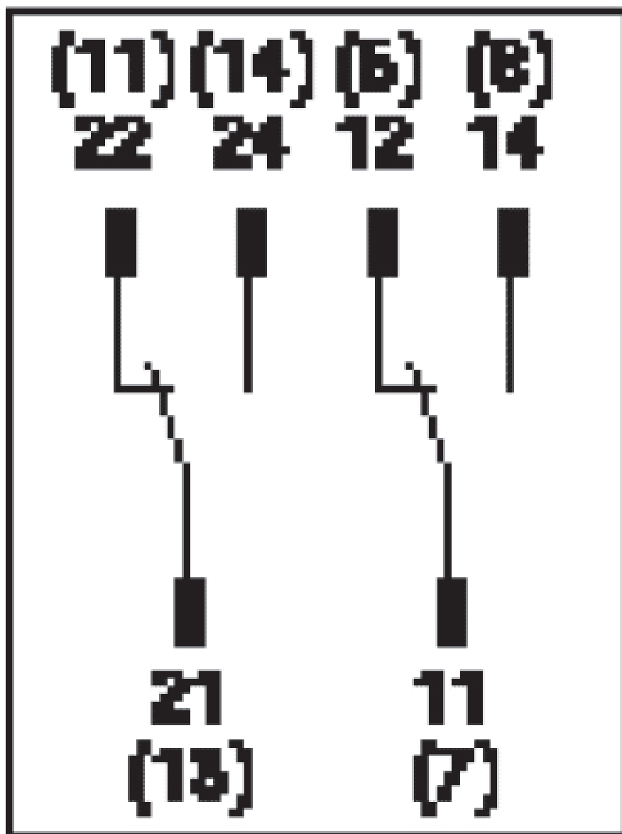
schakelschema
