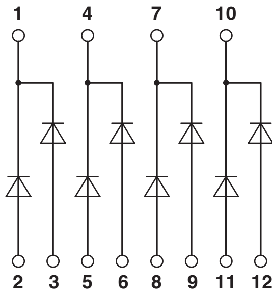
schakelschema
