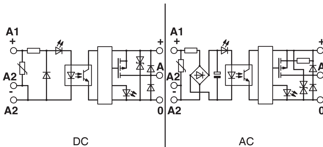
schakelschema
