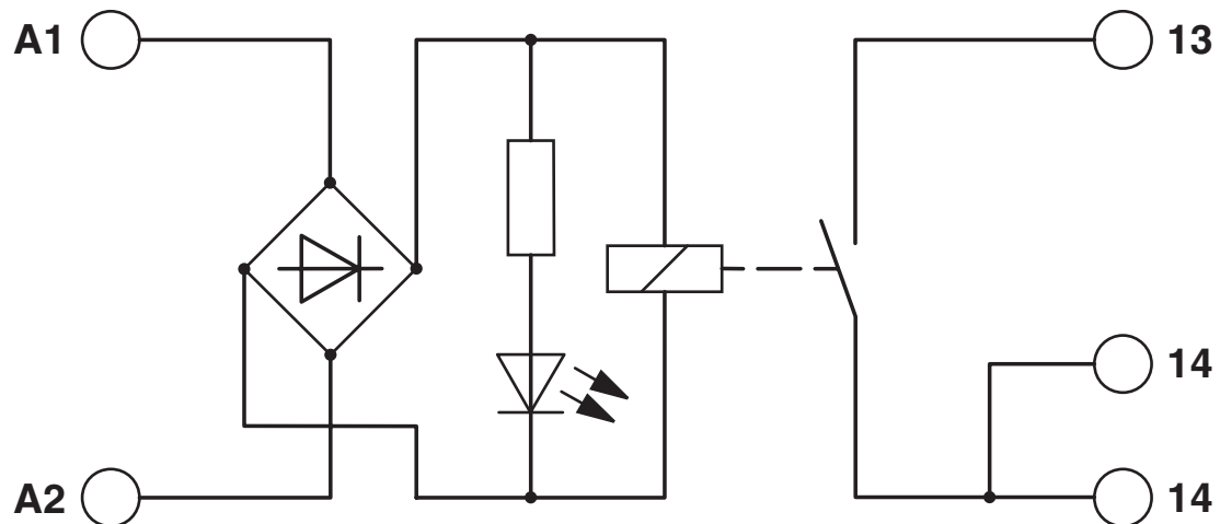
schakelschema
