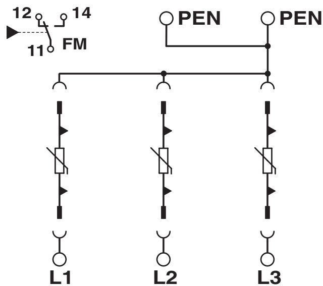
schakelschema
