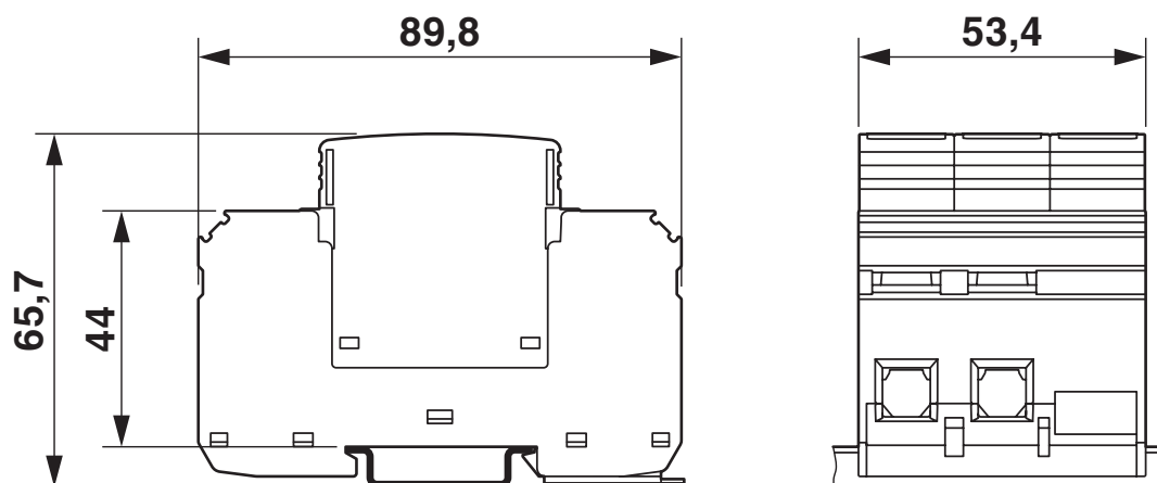
Maatschets
