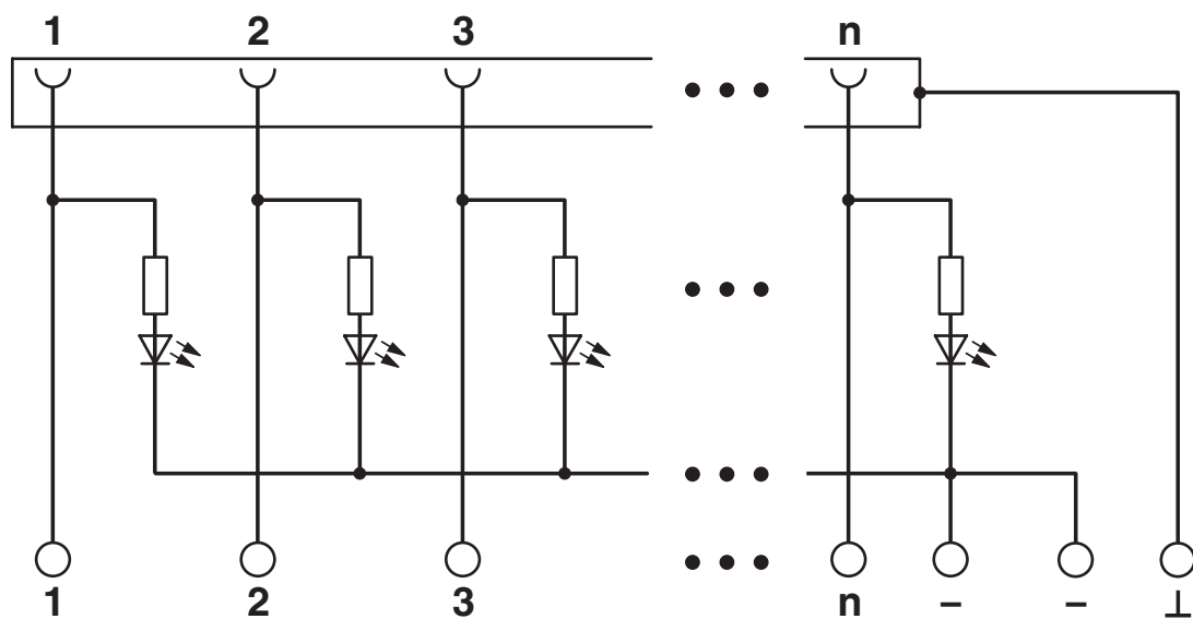
schakelschema
