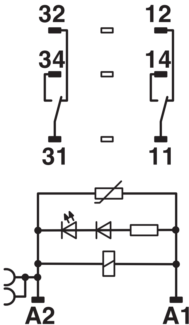
schakelschema
