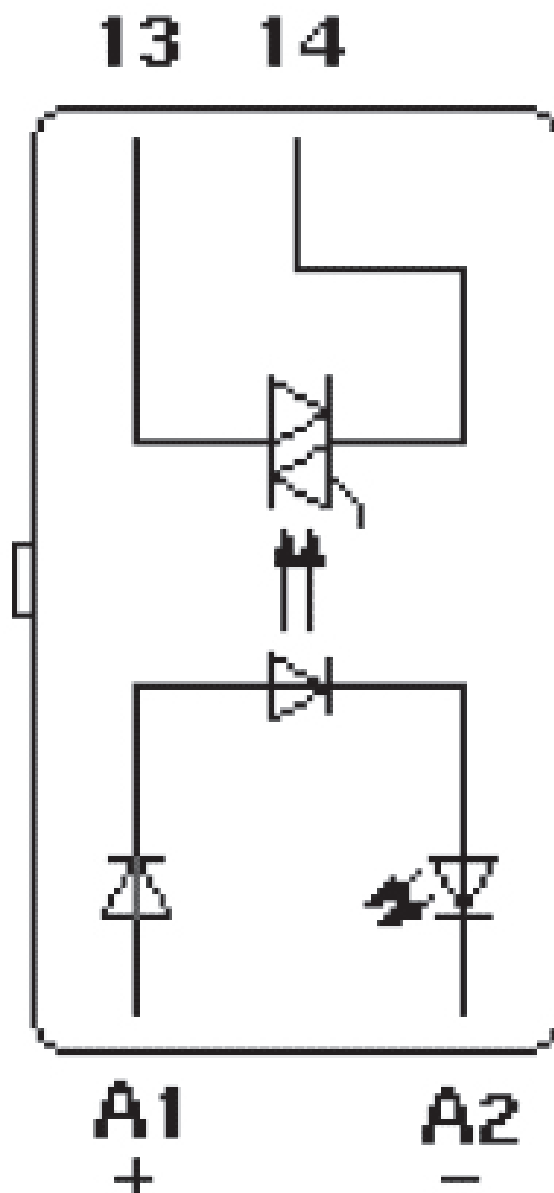
schakelschema
