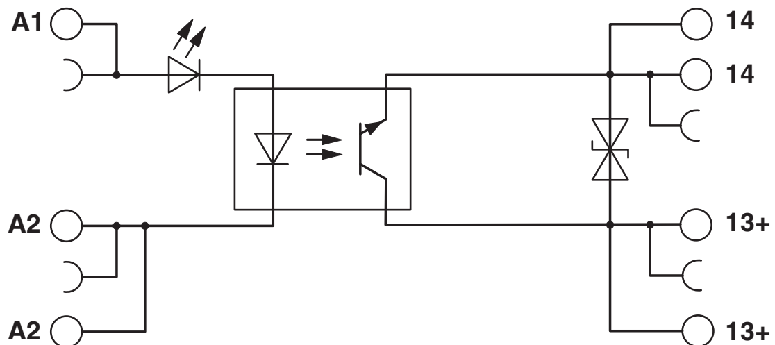
schakelschema
