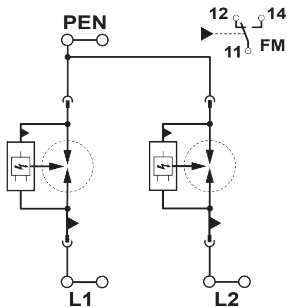
schakelschema
