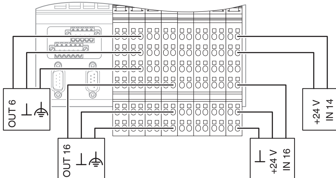
aansluitschema
