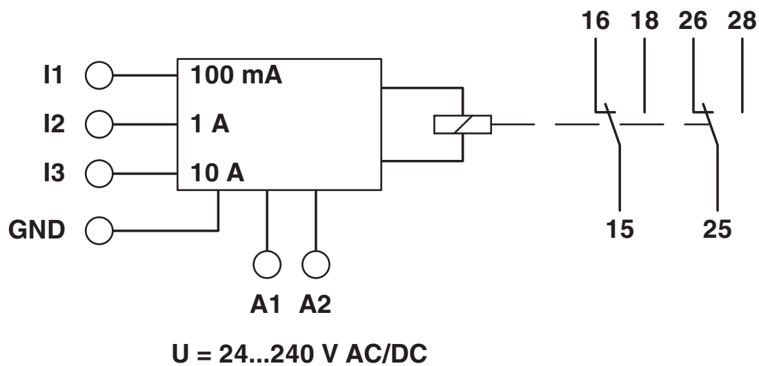
blokschema
