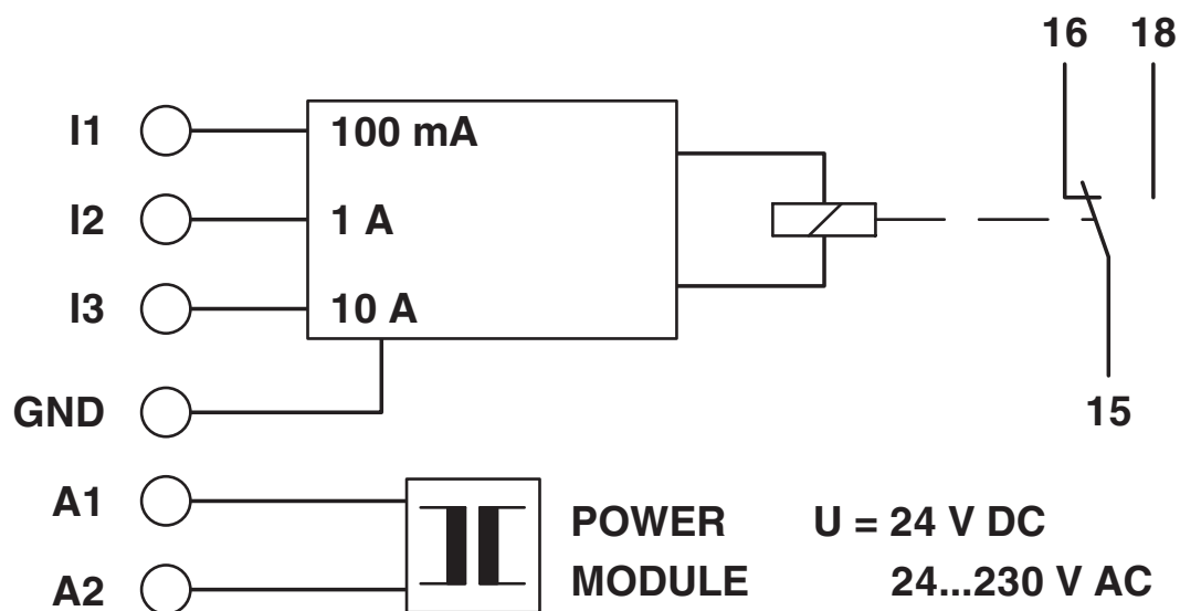
blokschema
