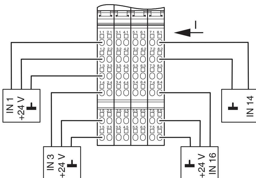
aansluitschema
