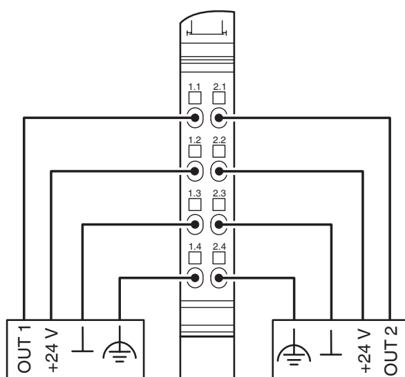
aansluitschema
