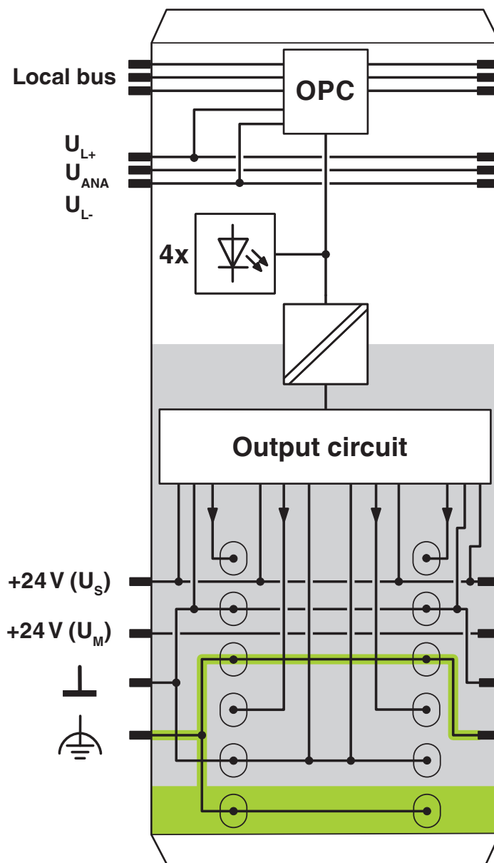
blokschema
