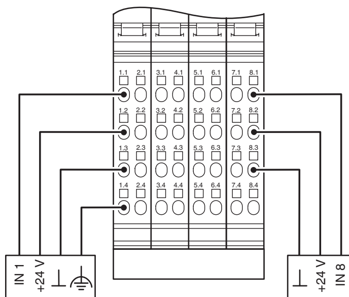
aansluitschema
