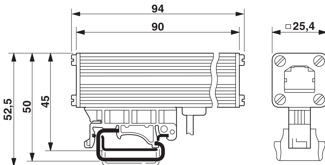
Maatschets
