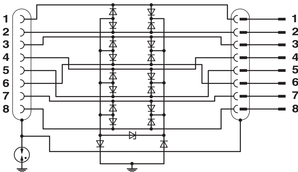
schakelschema
