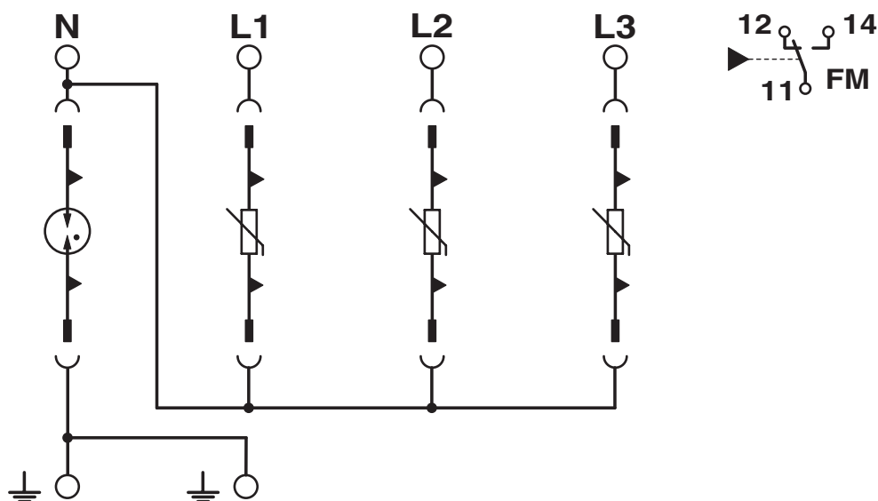
schakelschema
