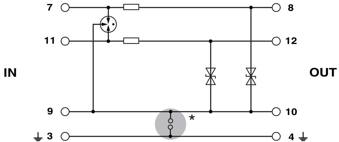
schakelschema
