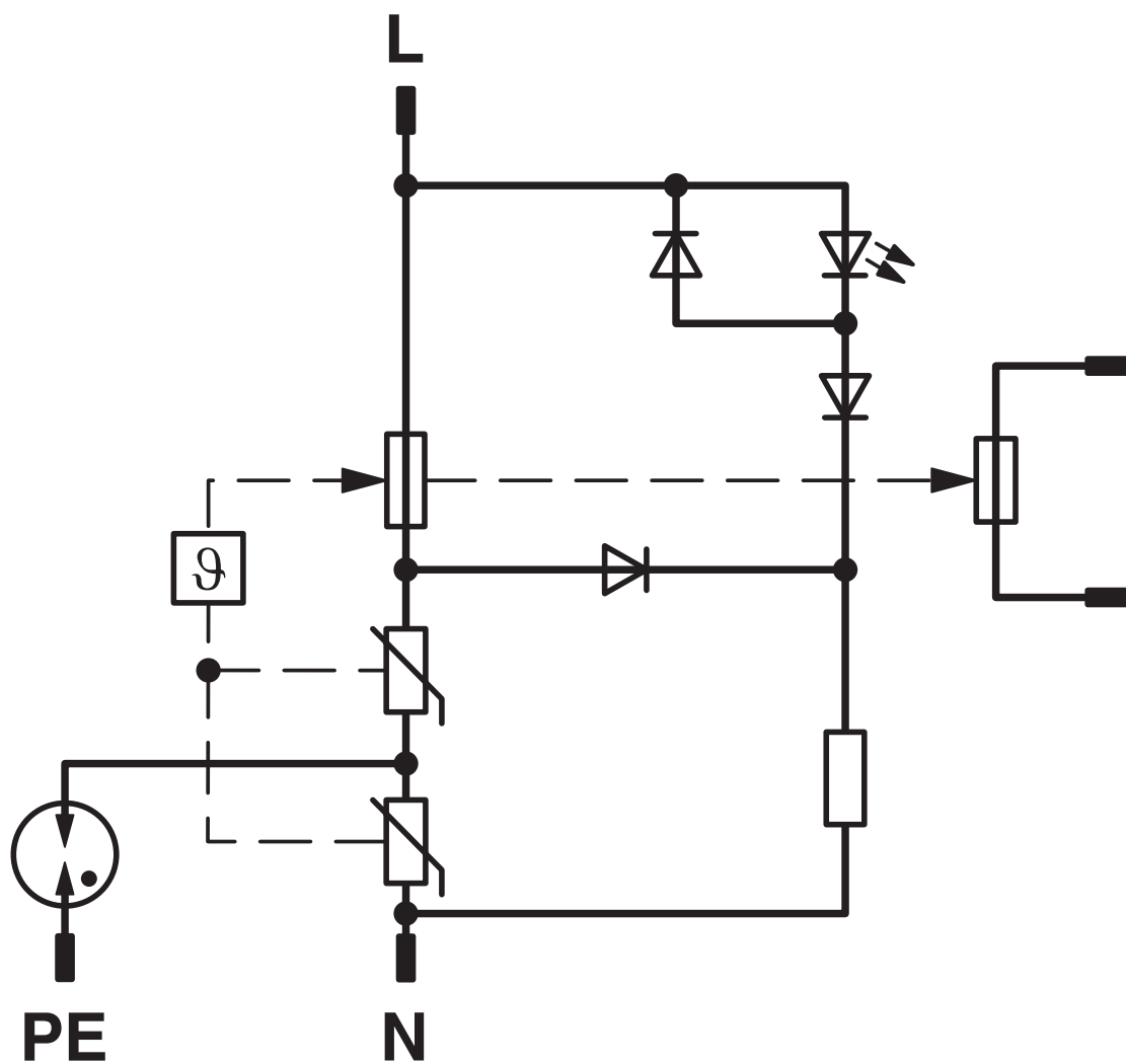
schakelschema
