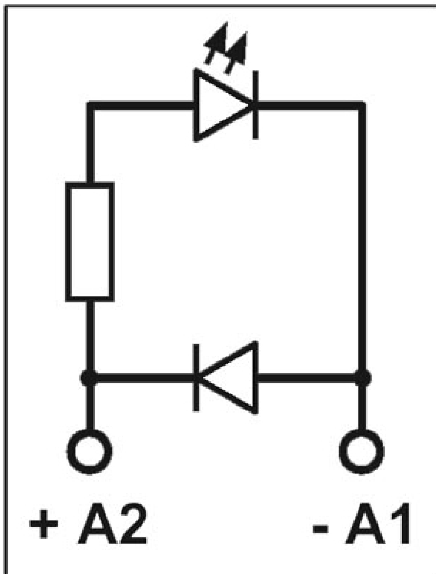
schakelschema
